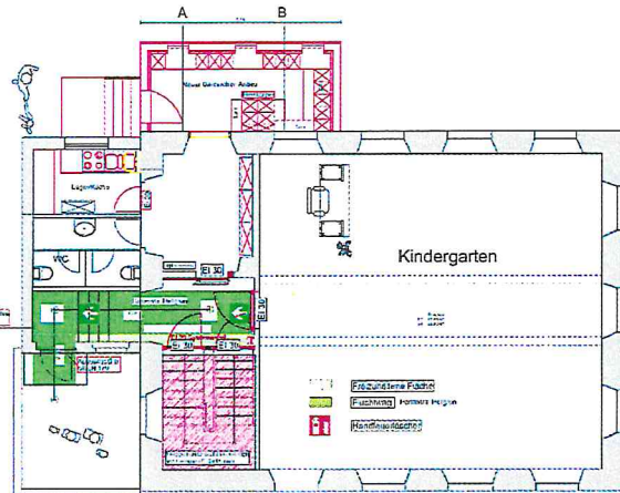
Abbildung 2: Aufsicht EG
